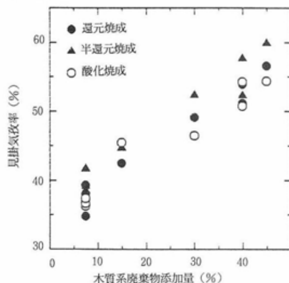
図2 木質系廃棄物添加量と見掛気孔率
