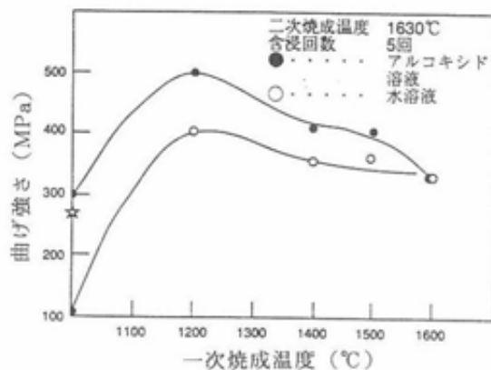
図8 一次焼成温度と含浸溶液による曲げ強さ
