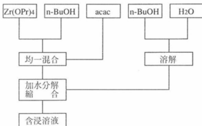
図4 アルコキシド溶液作製フロー
