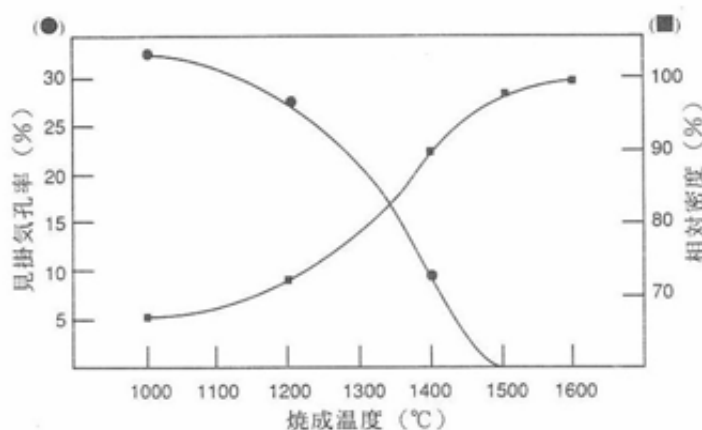
図2 焼成温度と見掛気孔率、相対密度
