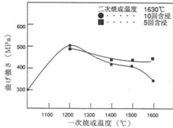
図7 一次焼成温度と含浸回数による曲げ強さ
