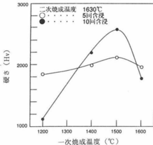
図10 一次焼成温度とビッカース硬度
