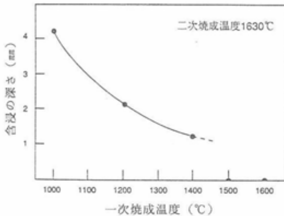
図5 一次焼成温度と含浸深さ
