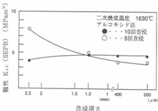
図9 含浸深さと靱性
