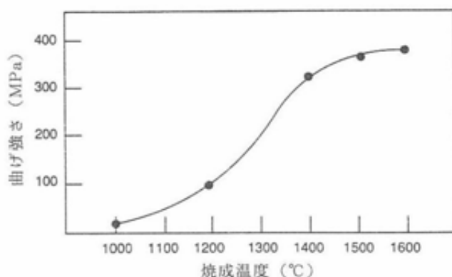
図3 焼成温度と曲げ強さ
