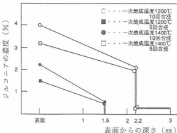
図6 含浸深さとジルコニアの濃度
