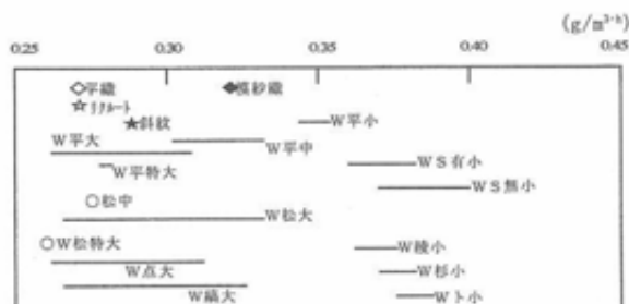
図17 組織・密度別の透湿度
