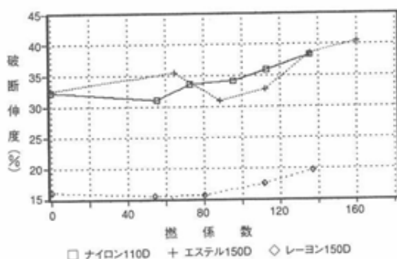
図3 各種フィラメントにおける撚係数と破断伸度との関係
