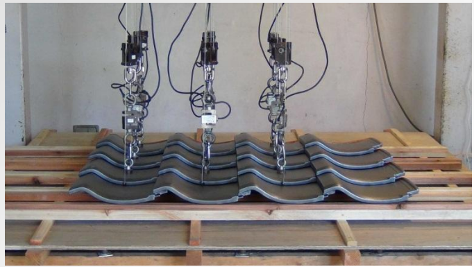
耐風圧性能試験
