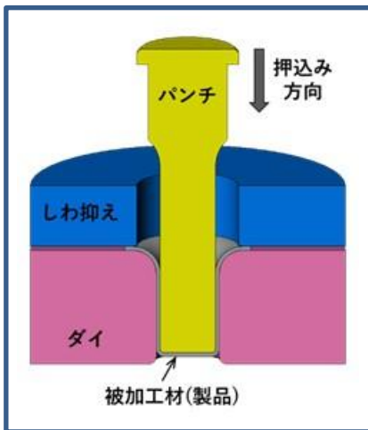
図 1 金型のモデル図
