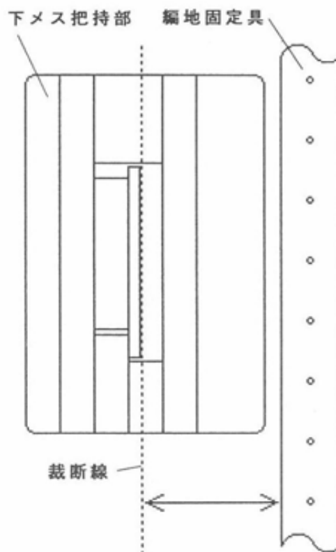
図5 下メス把持部と横編地固定具
