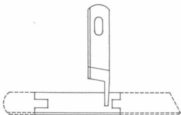
図3 上メス及び下メスの配置
