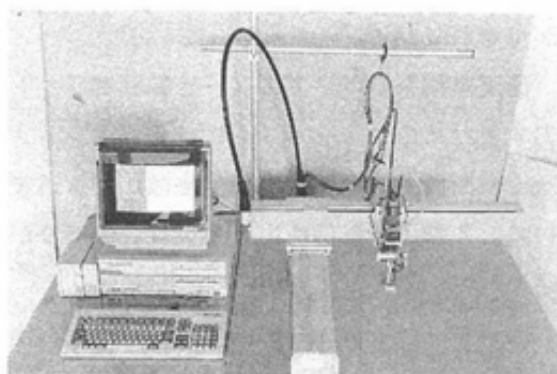
図8 横編地自動裁断装置
