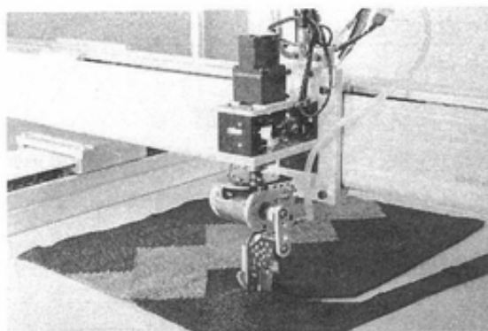
図9 裁断中のカッターヘッド
