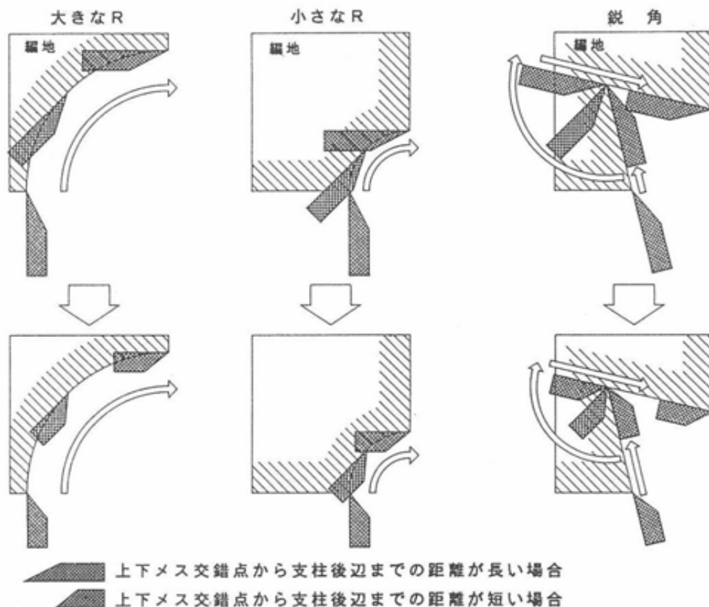
図1 メスの接触範囲
