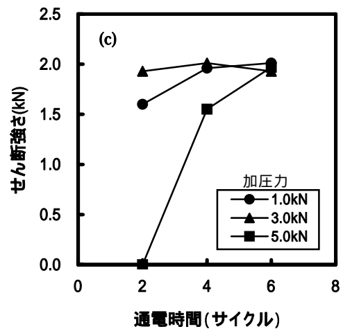
図 2 せん断試験結果
