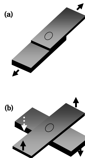
図1 接合強度用試験片の形状 (a)せん断試験片, (b)十字引張試験片
